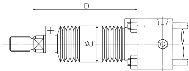
■寸法表[ネオプレン(J)・コーネックス(JC)]
