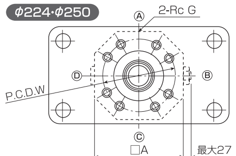
■FA形基本寸法表 [□はスイッチなし、スイッチ付仕様(φ80迄)の共通範囲です]
