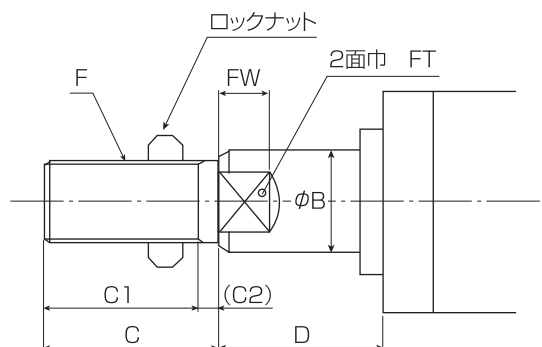
ロックナット付推奨ねじ長さ寸法
