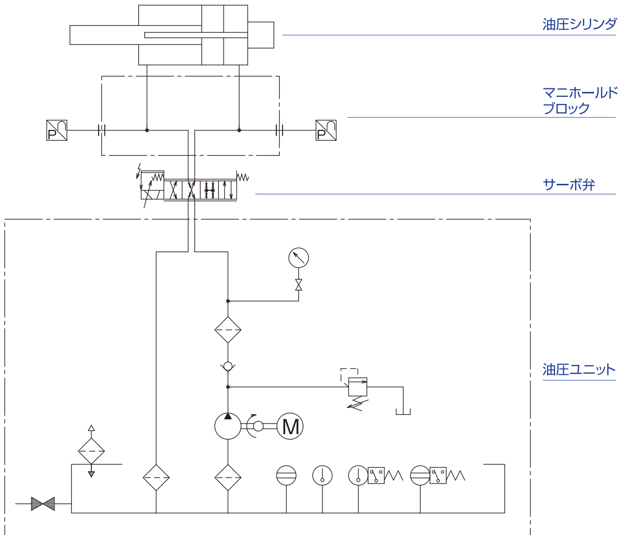
油压回路 (参考)
