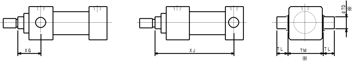
中間トラニオン形シリンダ (TC形)
