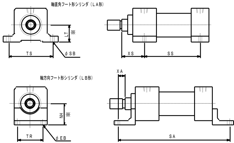
ロッド側長方形フランジ形シリンダ (FA形) 及び、ヘッド側長方形フランジ形シリンダ (FB形)
