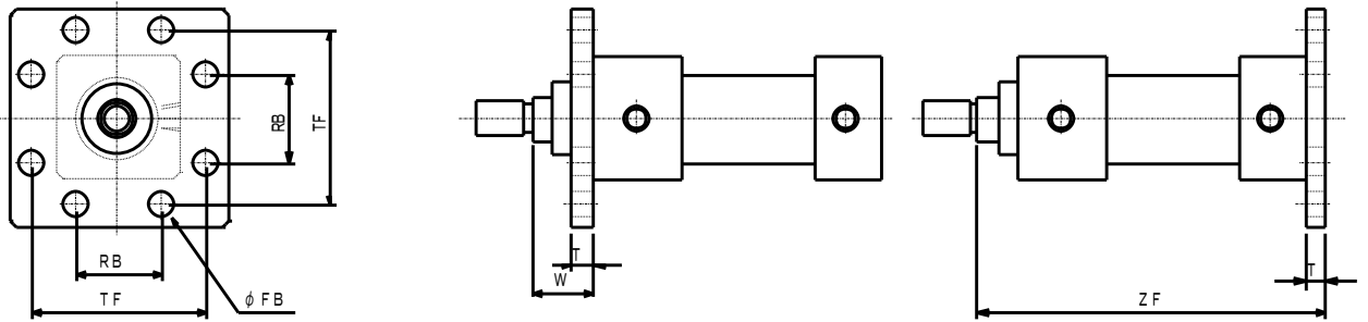
一山クレビス形シリンダ (CA形) 及び、二山クレビス形シリンダ (CB形)
