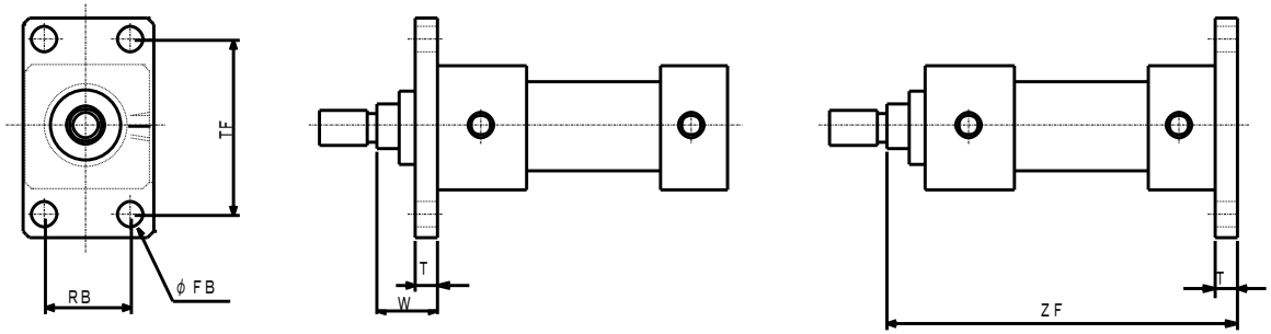
ロッド側正方形フランジ形シリンダ (FC形) 及び、ヘッド側正方形フランジ形シリンダ (FD形)
