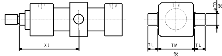
中間トラニオン形シリンダ (TC形)
