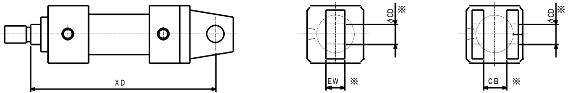
ロッド側トラニオン形シリンダ (TA形) 及び、ヘッド側トラニオン形シリンダ (TB形)
