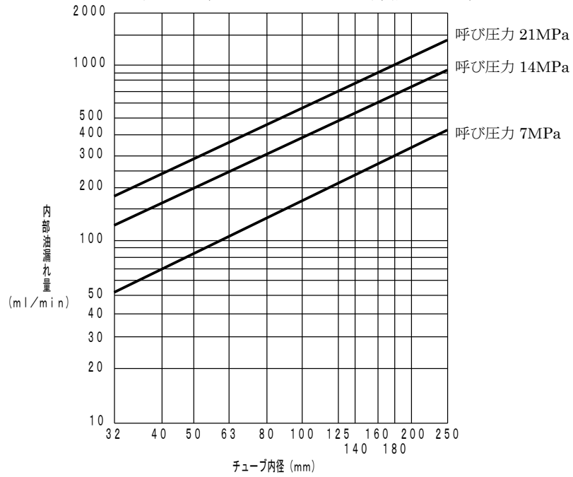
図4 (ピストンリング内部油漏れ量)
